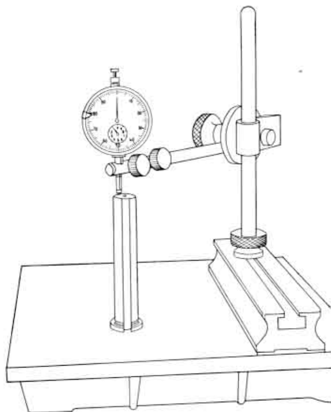
Fig. 18. - Azzeramento del comparatore sull'attrezzo A. 70037.
