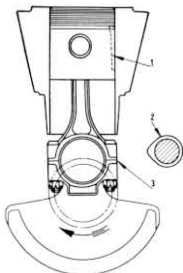
Fig. 6. - Mod. 500 L - 500 - 500 D e Nuova 500 Sport - Schema per il montaggio del complessivo biella-stantuffo sul motore. 1. Taglio di dilatazione - 2. Albero distribuzione - 3. Numerazione della biella.
