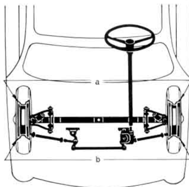
Fig. 21. - Mod. 500 - Schema per il controllo della convergenza ruote anteriori ( a - b = 0 \div 2 mm).
